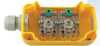
Art. SK2PM Original Mafelec Schaltkasten mit 2 Knöpfen: heben - senken 100 x 60 x 55 mm 78. 00 (F)
