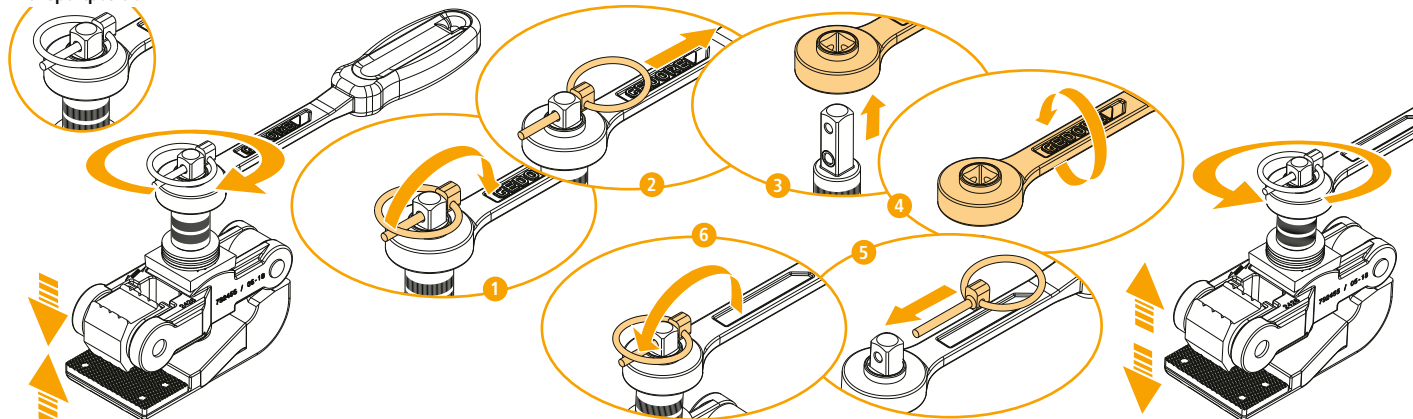
Bild 2 Schienenanschlussklemme mit abnehmbarer Ratsche
