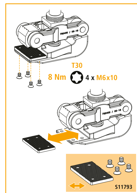
Bild 5 Austausch Kontaktplatte
