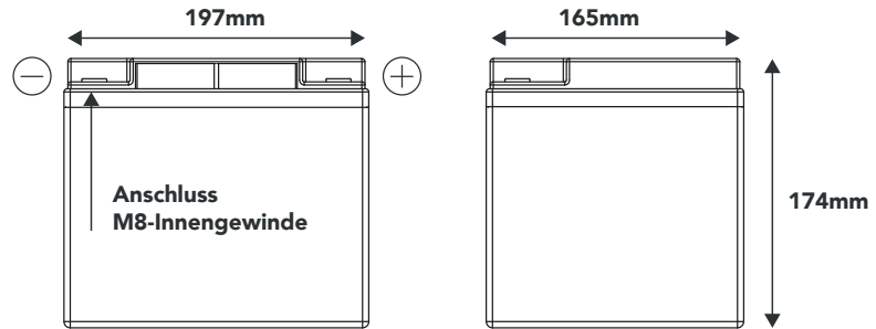
Abmaße: Länge 197mm | Breite 165mm | Höhe 174mm
