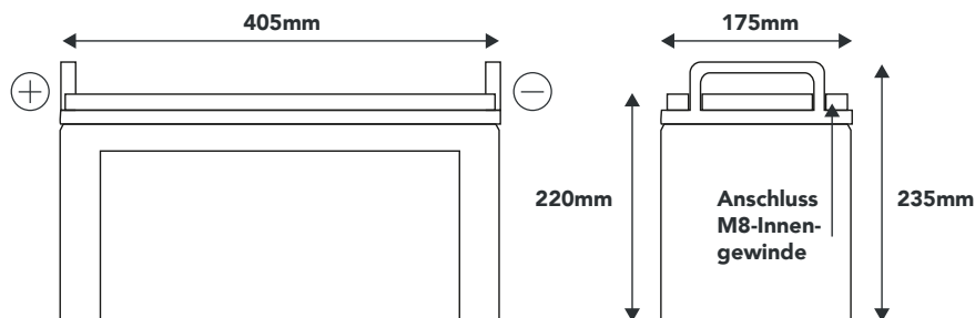
Abmaße: Länge 405mm | Breite 175mm | Höhe 235mm | Höhe ohne Griff 220mm
