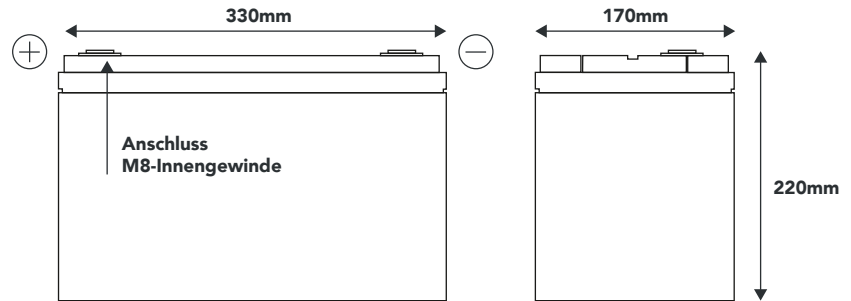
Abmaße: Länge 330mm | Breite 170mm | Höhe 220mm
