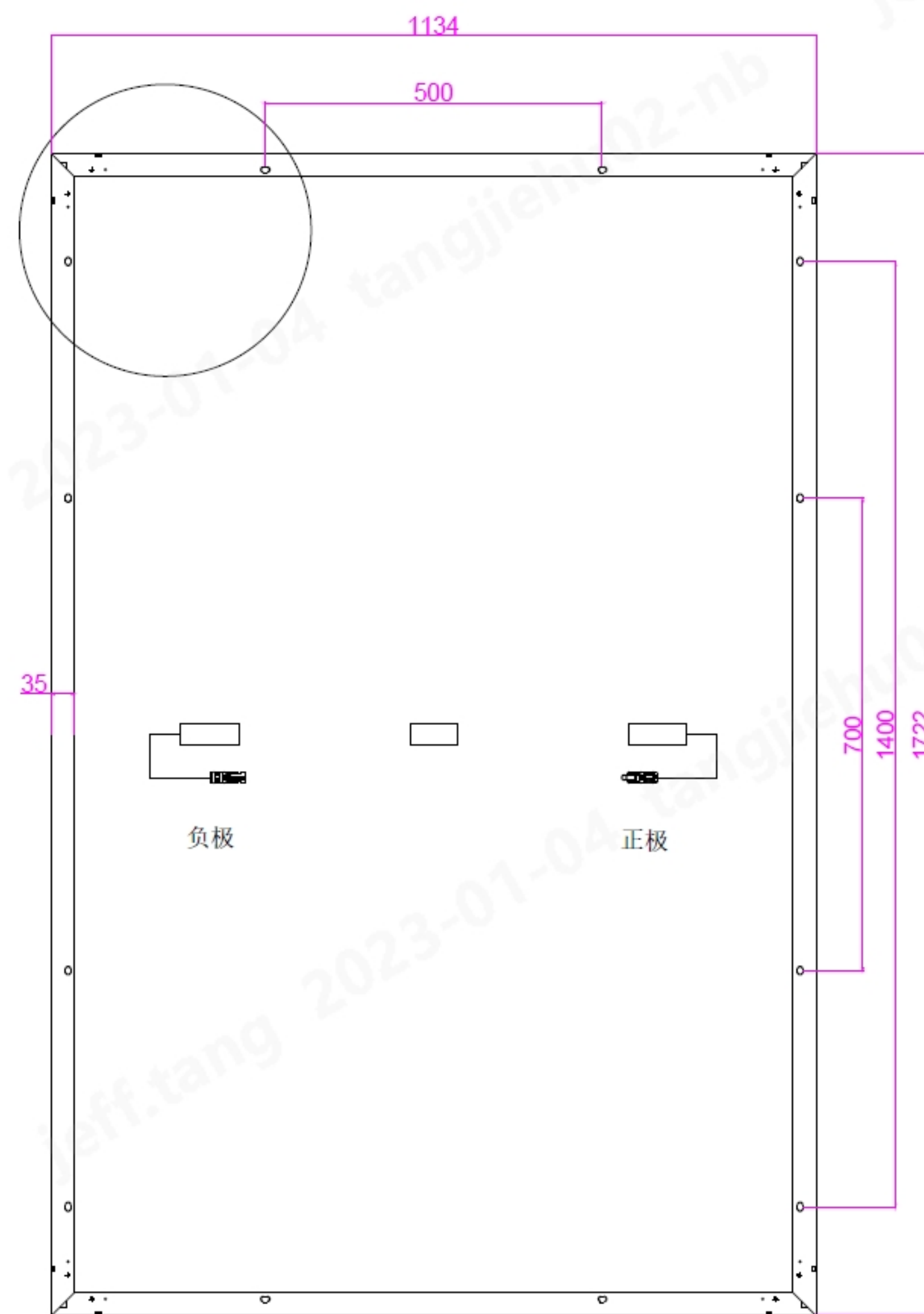
背面
