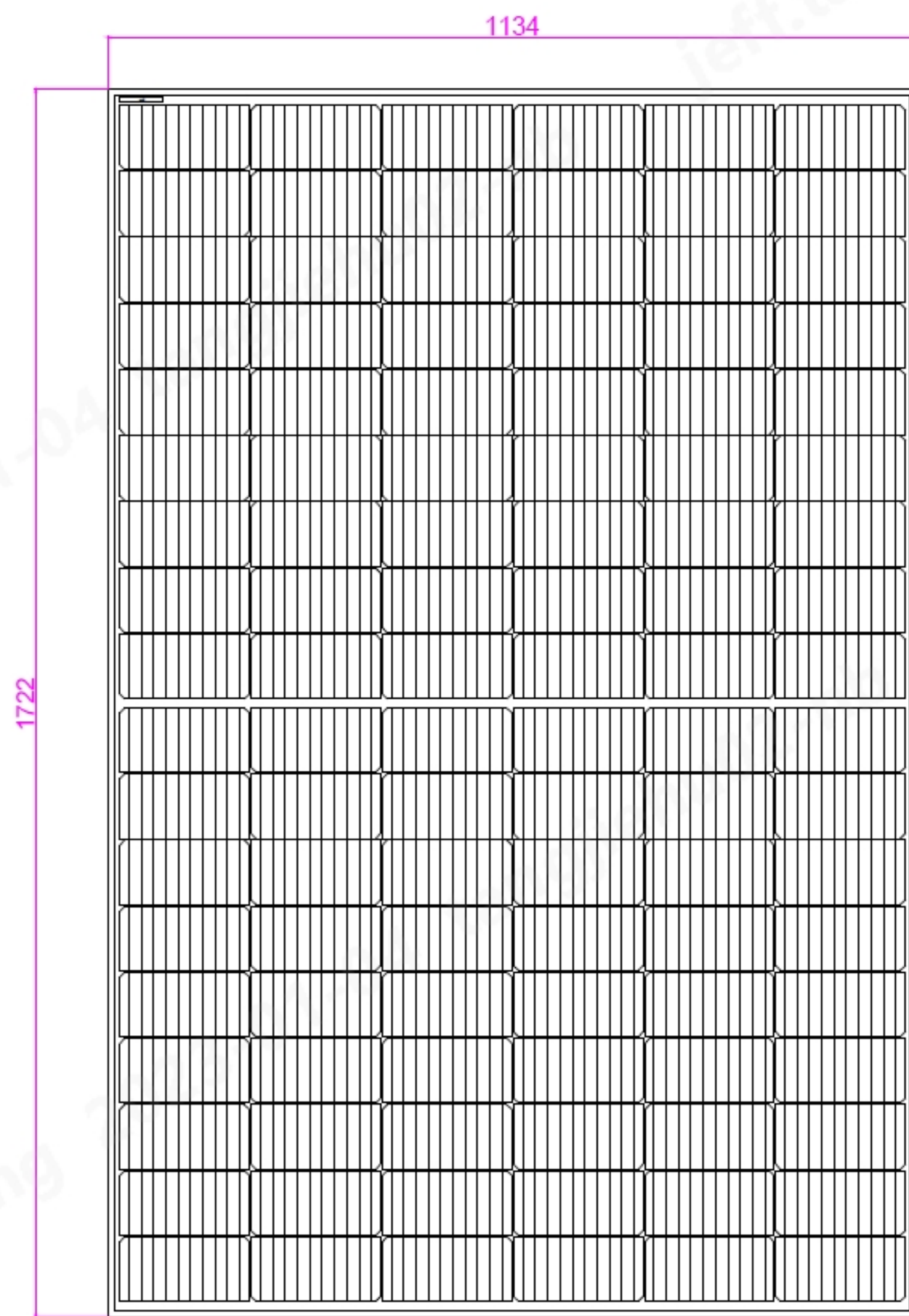
正面
