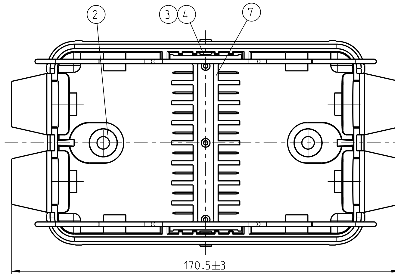
Ansicht ohne Deckel
