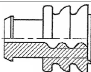
Bild zeigt Kontakt mit Einzelerdichtung Picture shows contact with single wire seal
