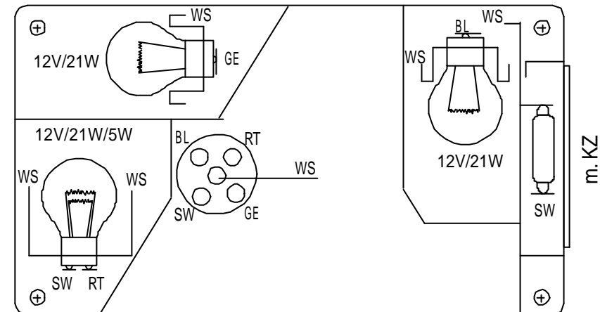
Ansicht Leuchte innen
