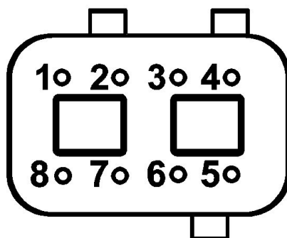
Pinbelegung, Ansicht von unten
