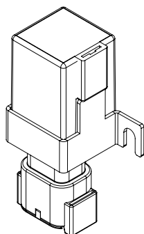
Einbauansicht mit Montagebügel
